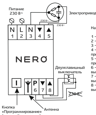
Рис. 1 — Подключение Radio 8113 micro
